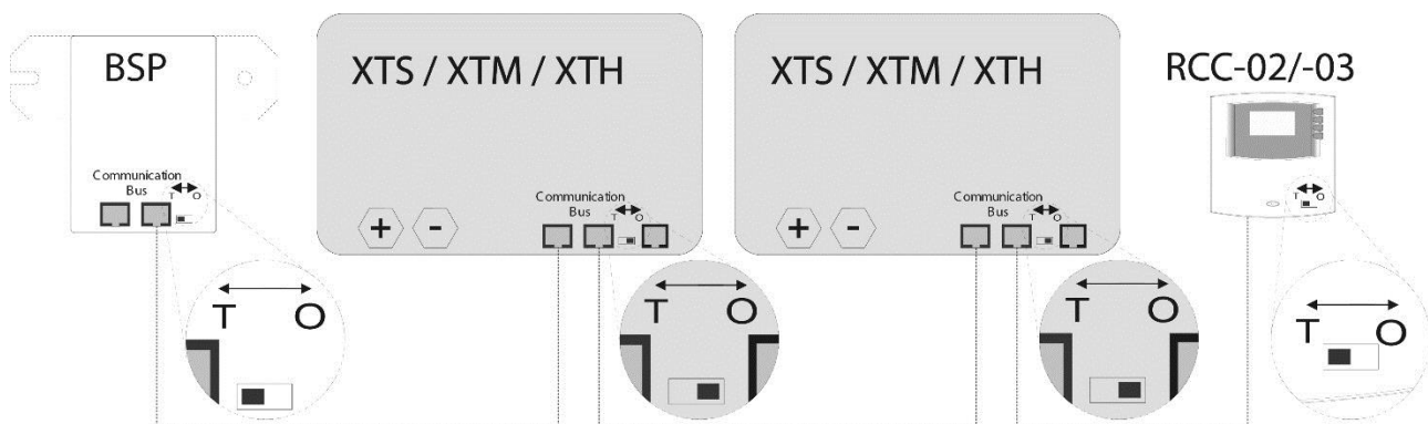
Ejemplo de una instalación con las terminaciones indicadas
