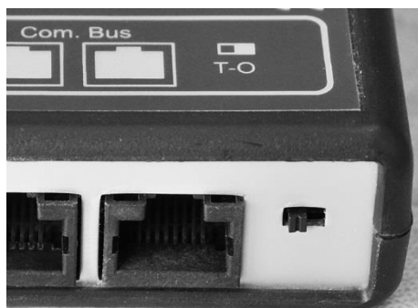
Terminación Xcom-232i activada (posición T)
