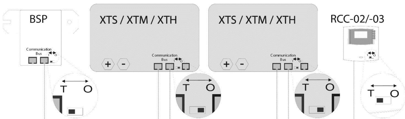
Installationsbeispiel mit der Korrekten Terminierung
