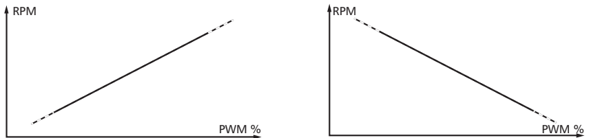
Abb. 6: Charakteristiken von Hocheffizienzpumpen mit PWM-Profil einer steigenden (AA, links) und einer fallenden Kennlinie (Ab, rechts)
